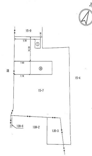
配置図
